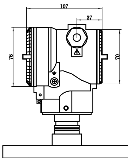
法兰侧面
