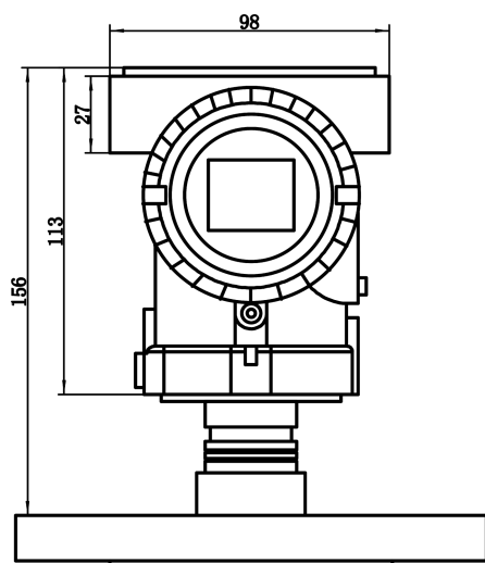
法兰正面
