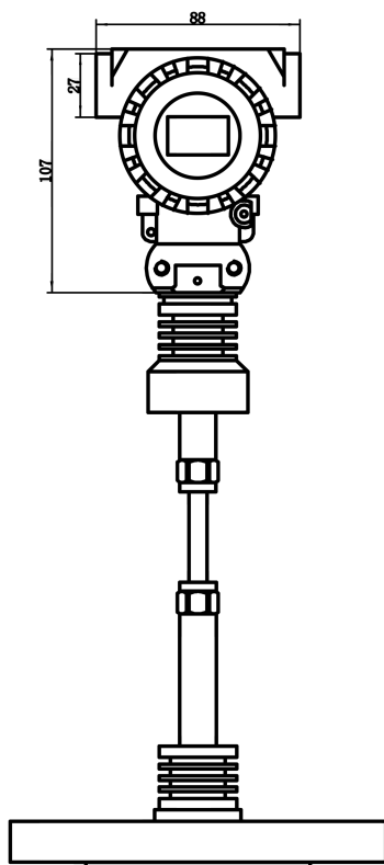
TS211-F法兰毛细管正面
