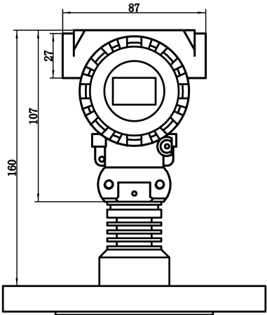
TS211-F法兰正面
