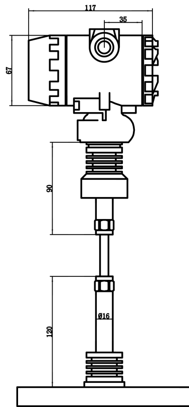
TS211-F法兰毛细管侧面
