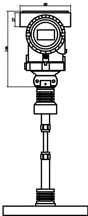
TS211-TG法兰毛细管正面
