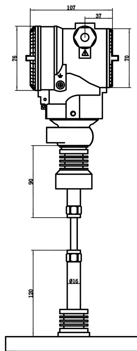
TS211-TG法兰毛细管侧面
