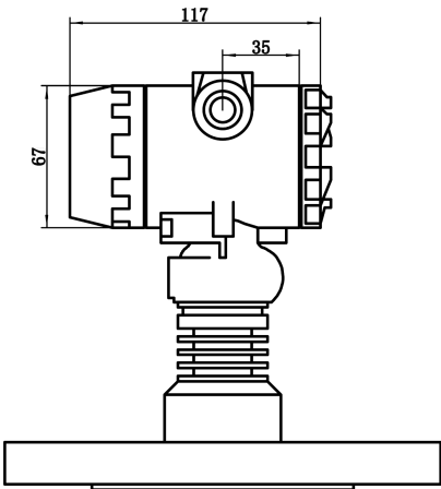
TS211-F法兰侧面
